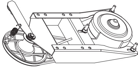
Привод двери F012.200-52
