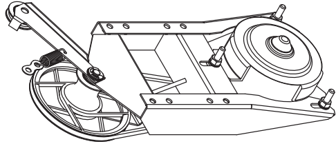
Привод двери Г012.200-54
