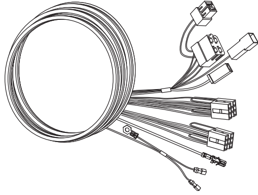
Жгут основной Г012.050-01 (ГАЗель Бизнес)
