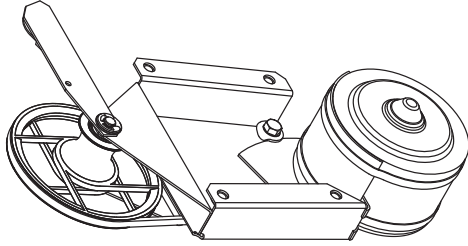
Привод двери Г016.200
