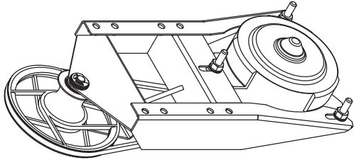
Привод двери Г012.200-53
